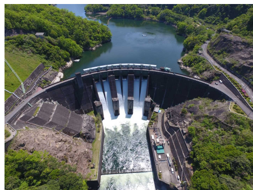
非常用洪水吐からの放流 （令和元年5月のフラッシュ放流）
