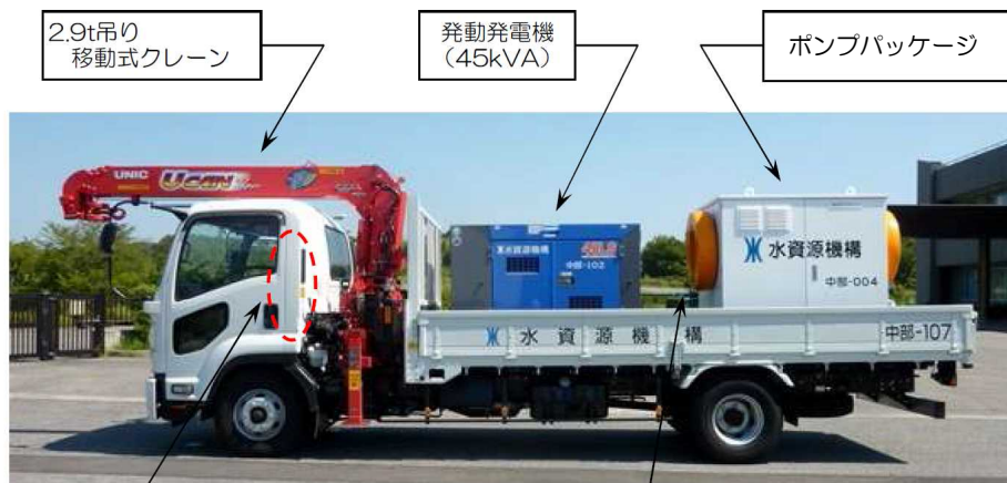
【ポンプパッケージ輸送状態】
