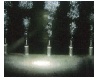
曝気循環設備の稼働状況(左:水面 右:吐出口)
