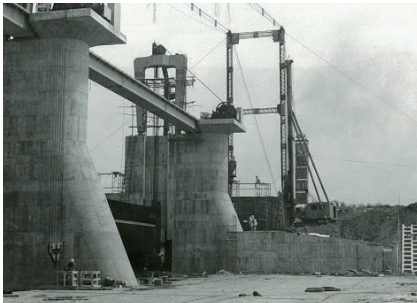
建設中の秋ヶ瀬取水堰
