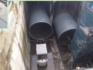
鋼管を設置した宗岡副水路
