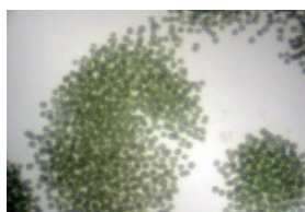
ミクロキスティス属
