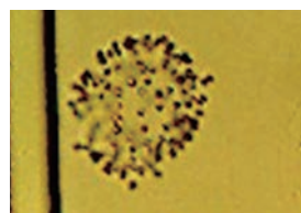
ウログレナ属
