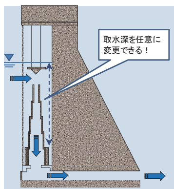
選択取水設備（イメージ図）
