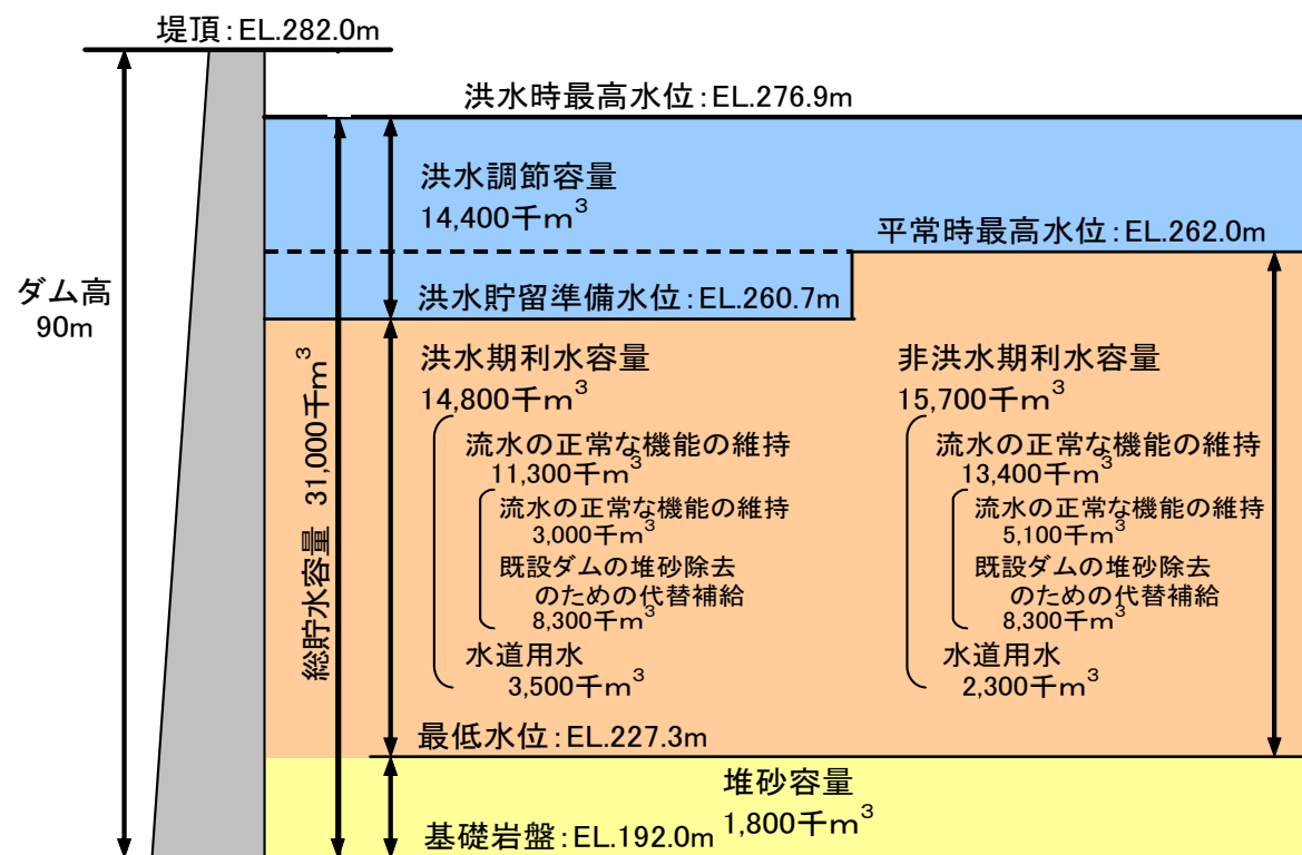
川上ダム貯水容量配分図
