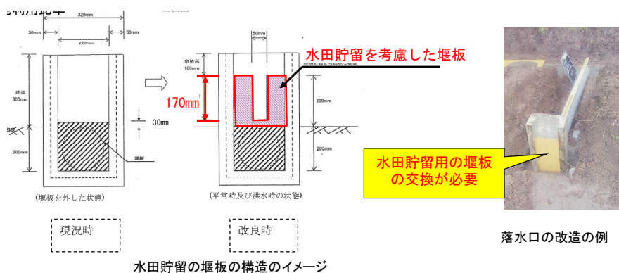
水田貯留の堰板の構造のイメージ
