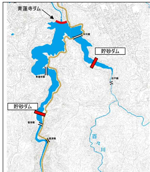
青蓮寺ダム 貯砂ダム候補地
