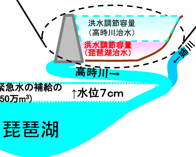
丹生ダム貯水池容量配分図(B案)
