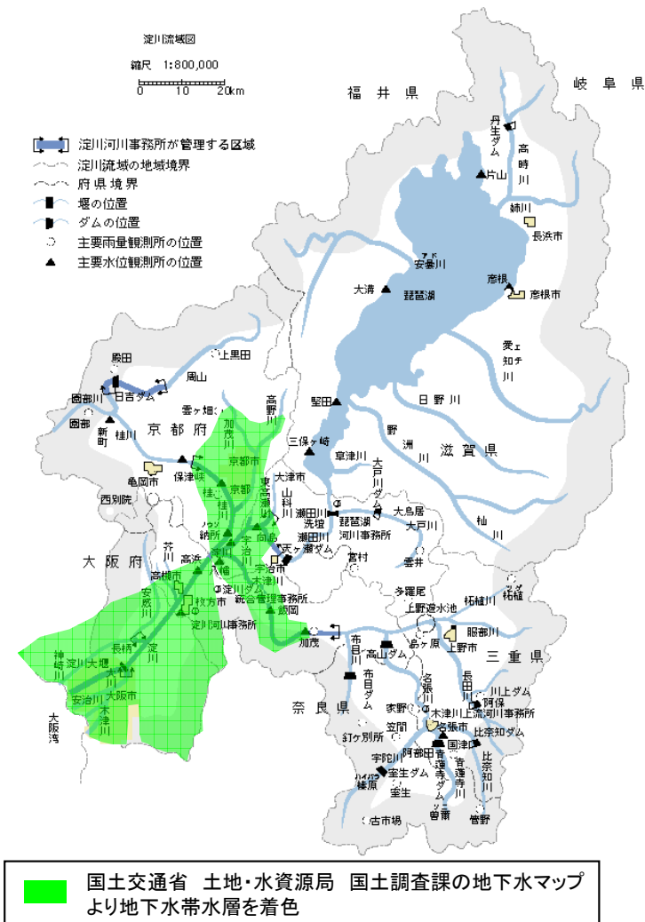
淀川流域の井戸の新設可能範囲
