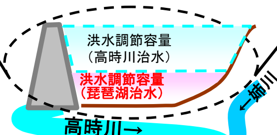
丹生ダム貯水池容量配分図(B案)
