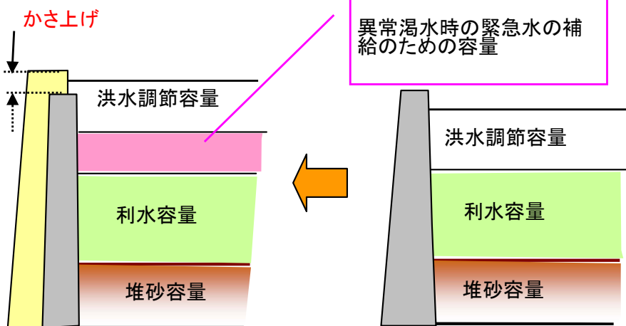
既設ダムかさ上げによる容量確保イメージ
