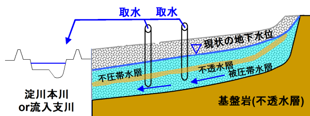
図 4.5.27 地下水取水イメージ
