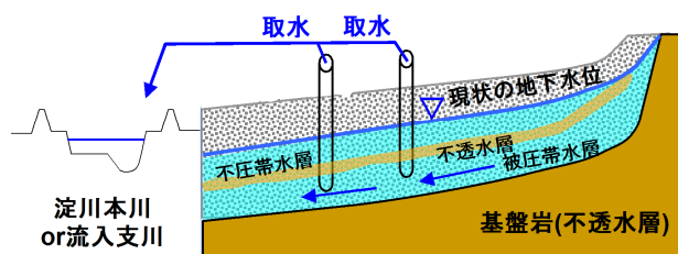
図 4.5.40 地下水取水イメージ
