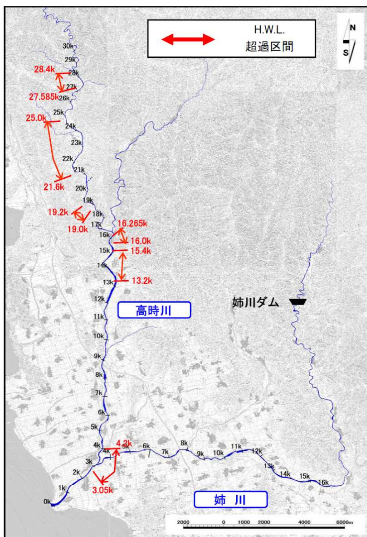
図 4.3.15 計画高水位 (H.W.L.)超過区間全体図
