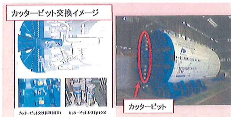
図35 カッタービット交換イメージ
