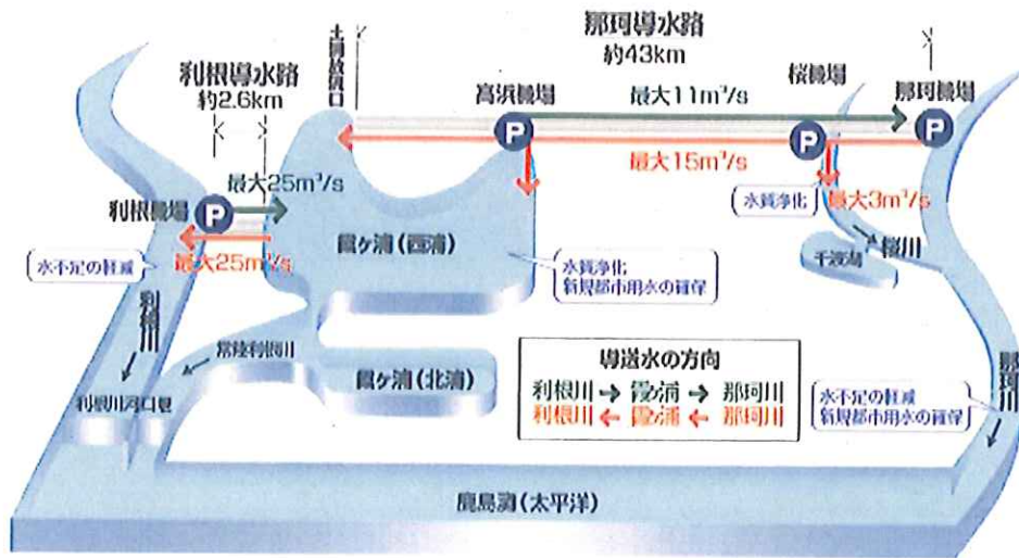
図7 霞ヶ浦導水の概要 (出典：霞ヶ浦導水工事事務所 HP)
