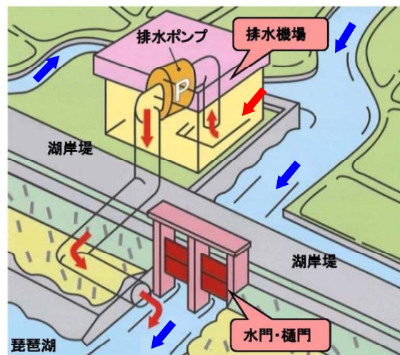
排水ポンプのはたらき
