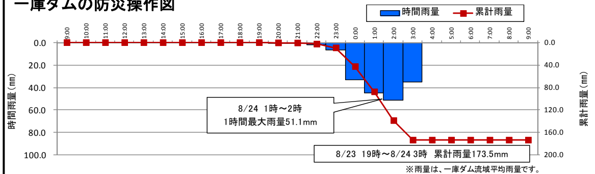
一庫ダムの防災操作図
