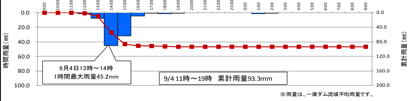
一庫ダムの防災操作図
