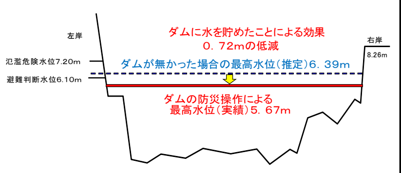
多田院地点における水位低減効果
