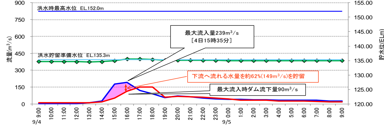
一庫ダムの防災操作図
