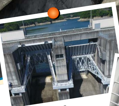
◎ 非常用洪水吐設備
