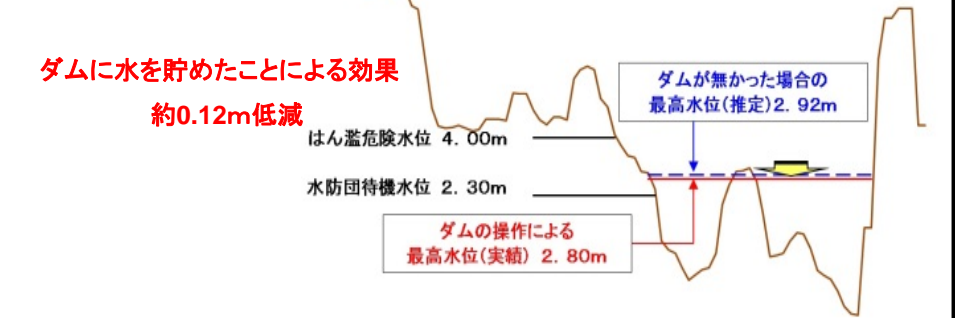
保津橋地点における水位低減効果
