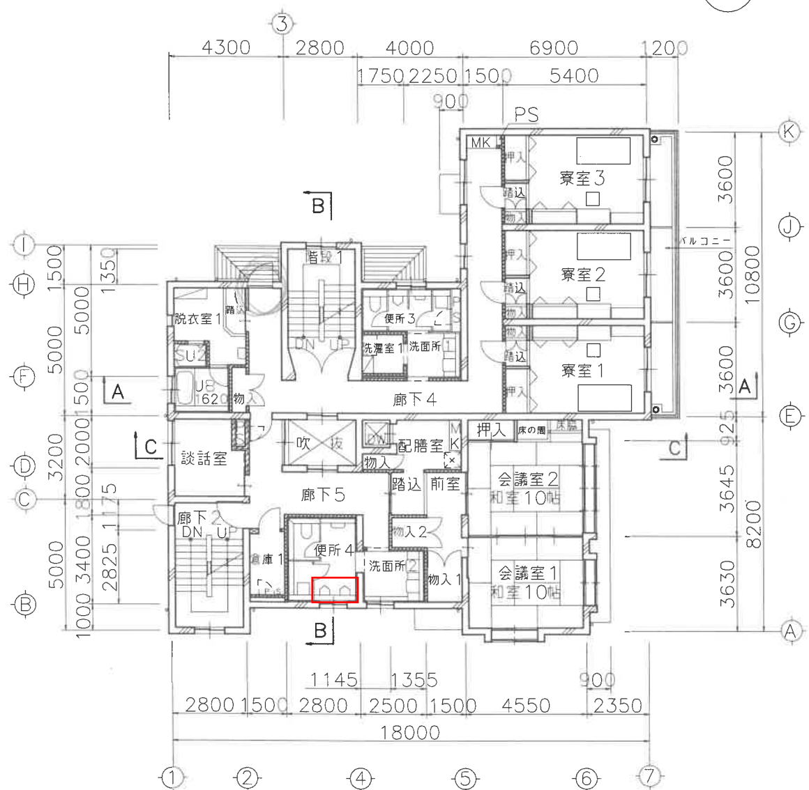
2 階平面図
