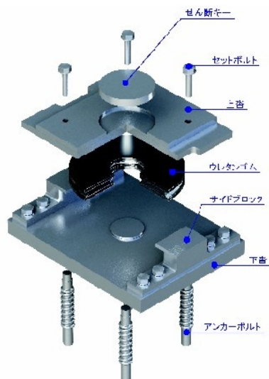
【当初設計】 反力分散支承
