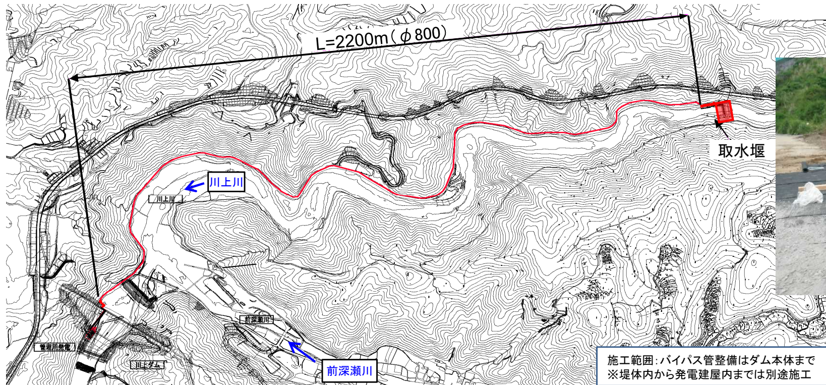
バイパス管施工状況
