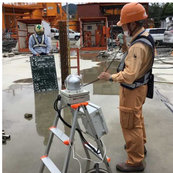
参考(Webカメラ地上設置状況)
