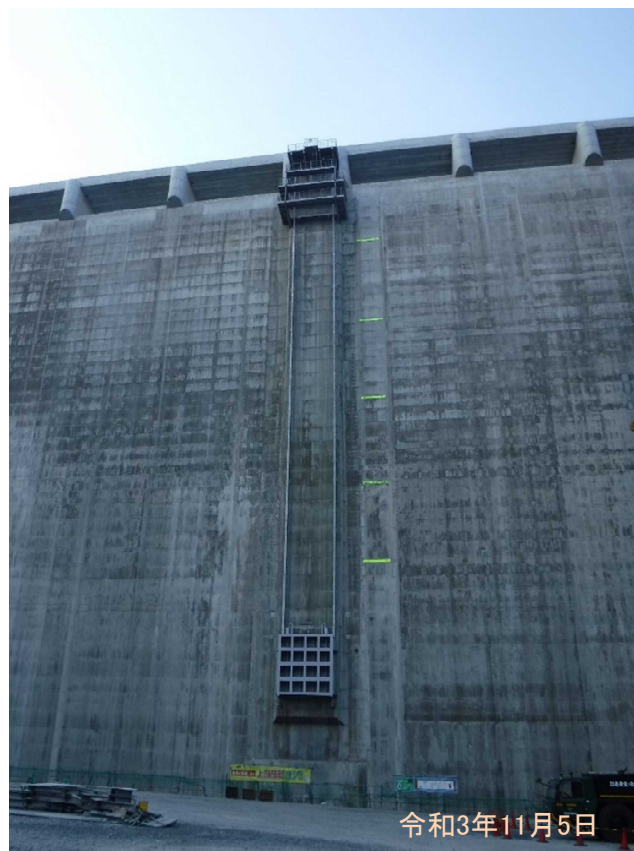
修理用ゲート設置状況
