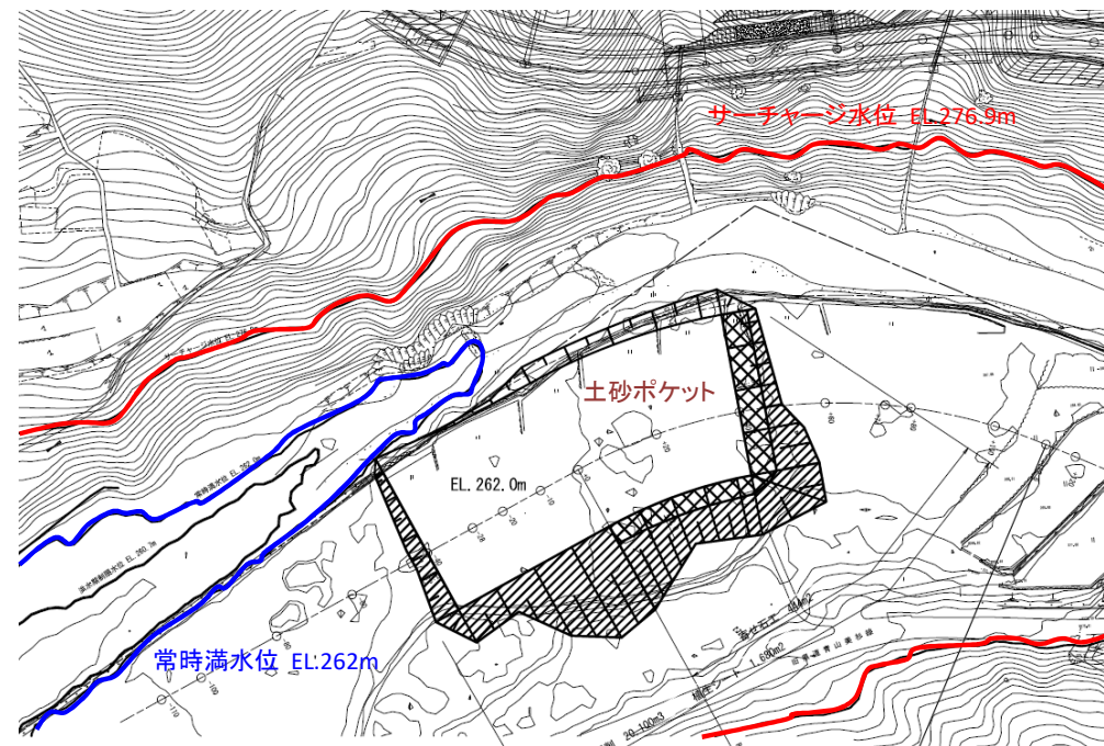
土砂ポケット平面図
