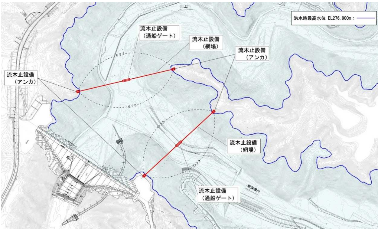
流木止設備平面図
