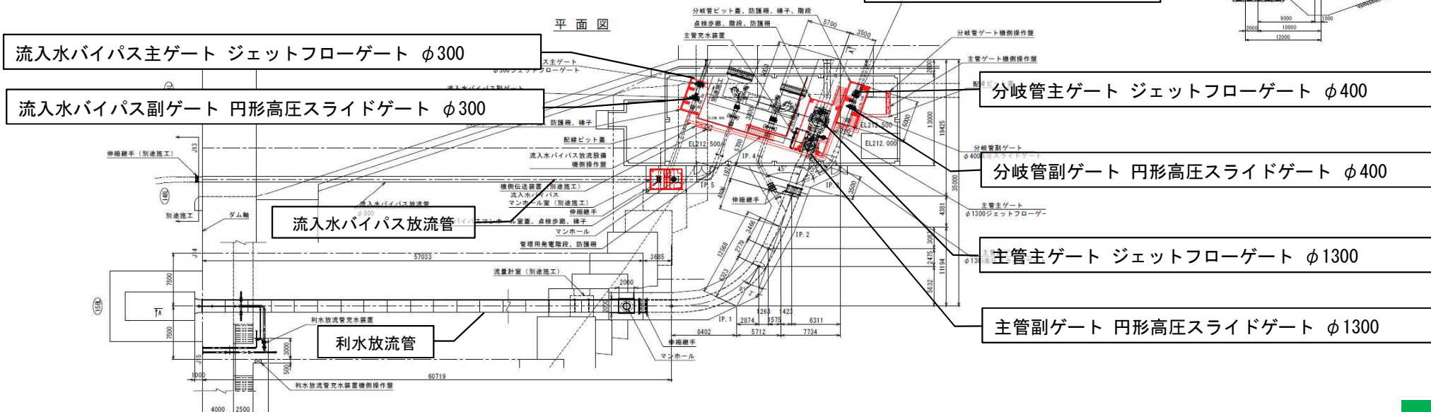
利水放流設備・流入水バイパス放流設備平面図
