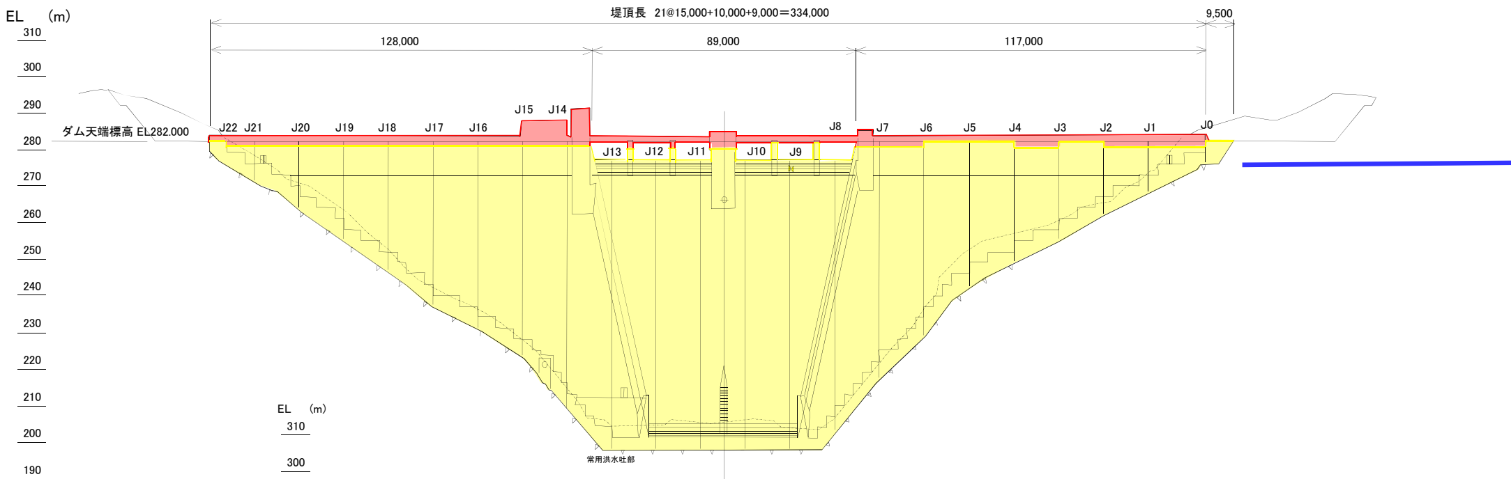
標準断面図
