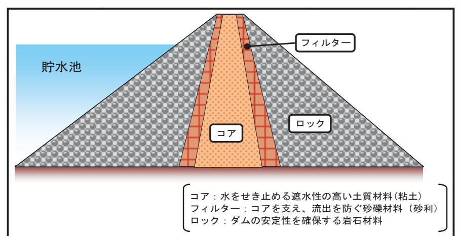
ロックフィルダムの構造
