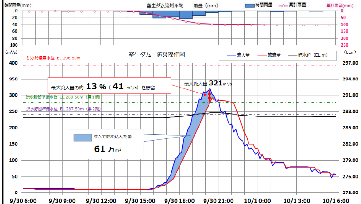
室生ダムの防災操作図
