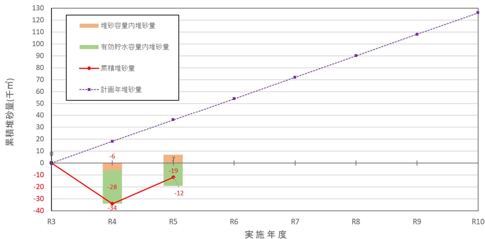
計画及び累積堆砂量 経年変化図
