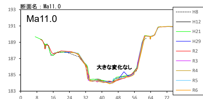
河床高の経年変化(断面図)
