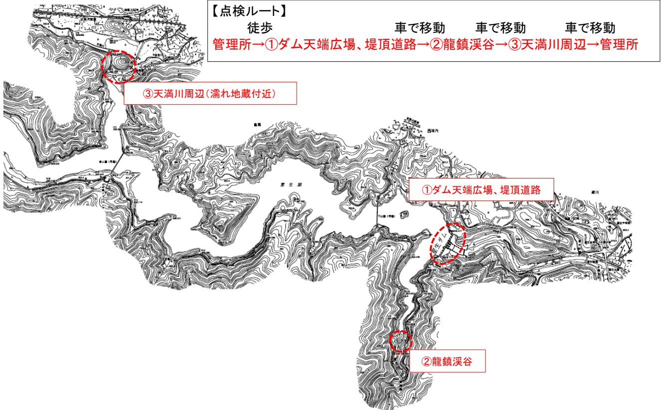
点検箇所図
