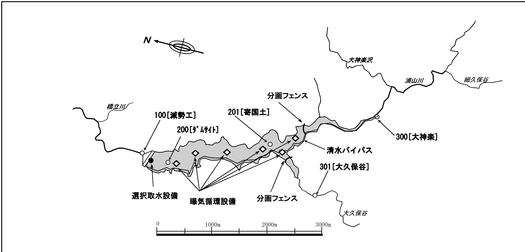
浦山ダムの水質調査位置図
