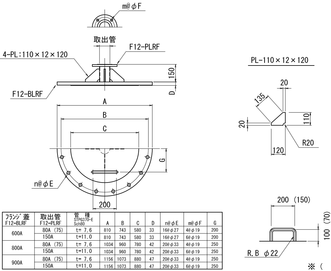
空気弁用フランジ蓋詳細図 (0.98Mpa) S=1:10
