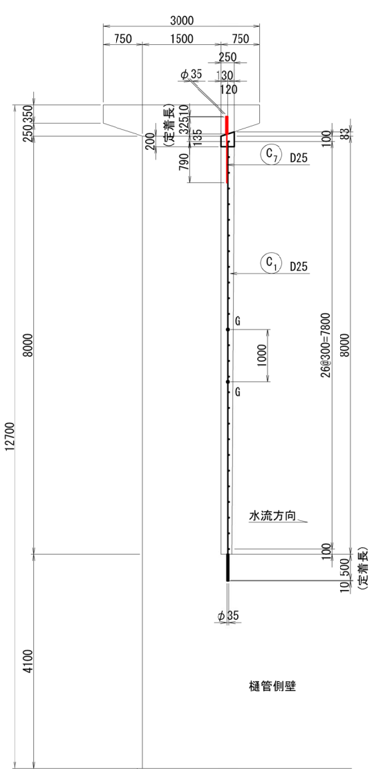
3 - 3 (側面図)
