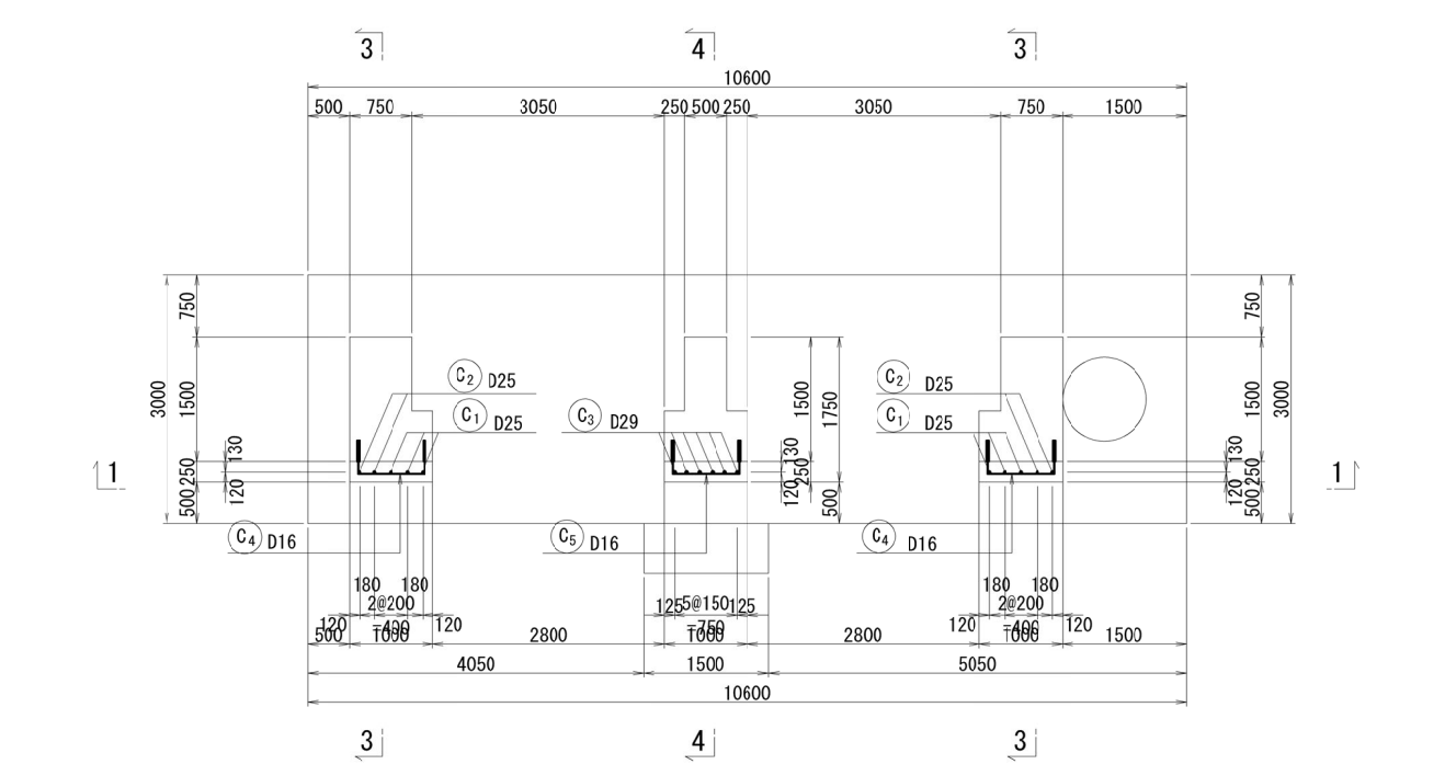
2 - 2 (平面図)
