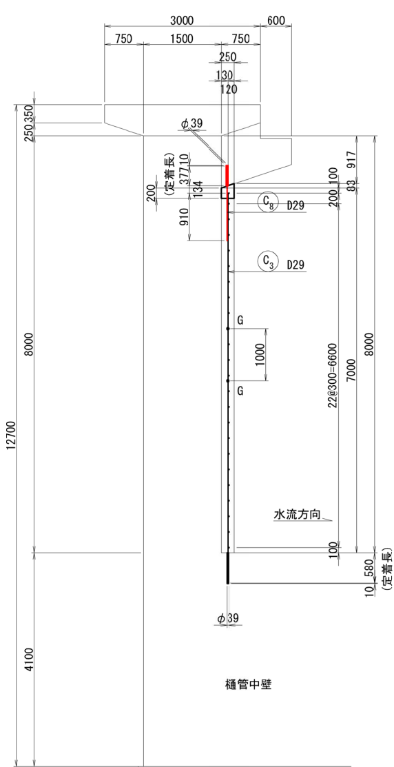
4 - 4 (側面図)
