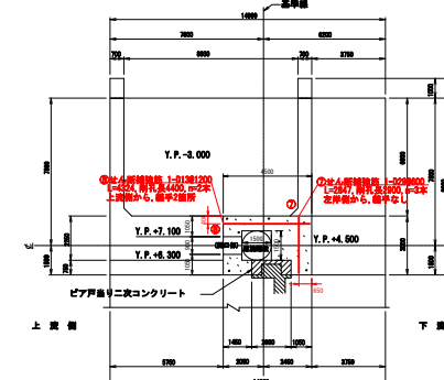
F-F断面
