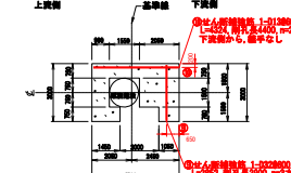
E-E断面
