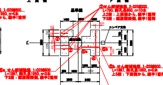
A-A断面
