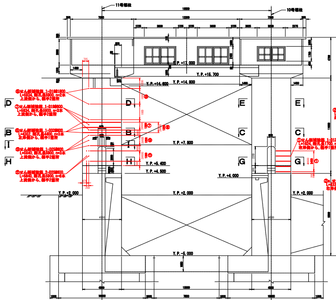
上流面
