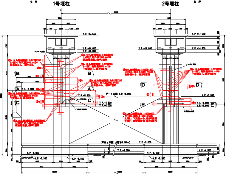
上流側
