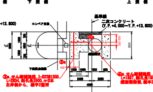
C-C断面
