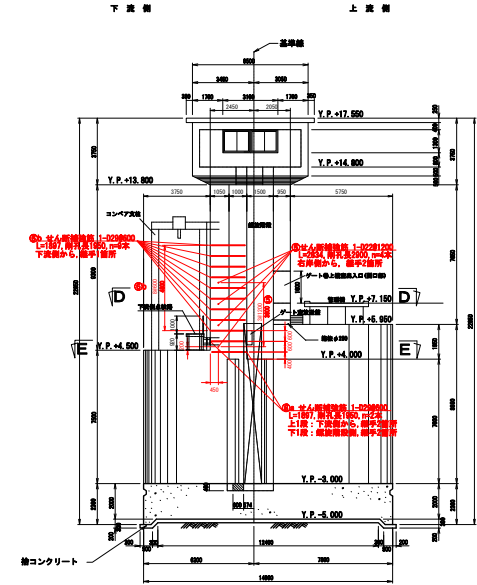
D-D断面
