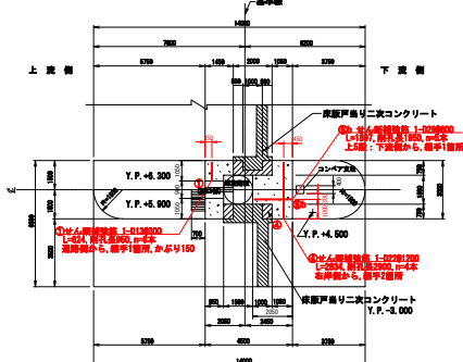
C-C断面
