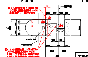
E-E断面
