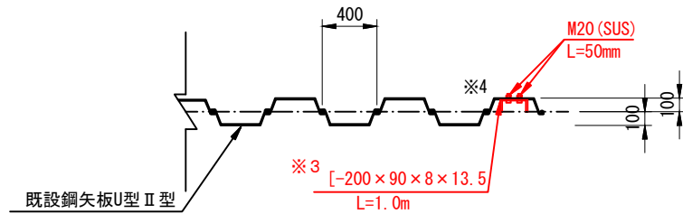
平面图 S=1:50
