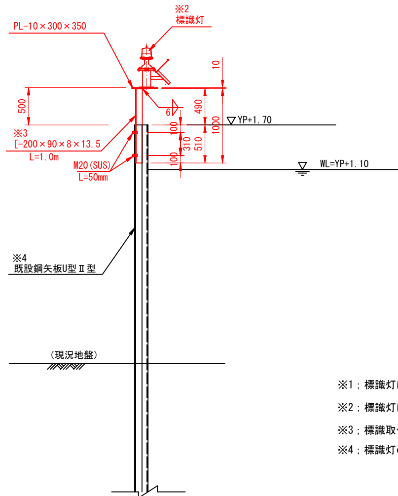
断面図 S=1:50
