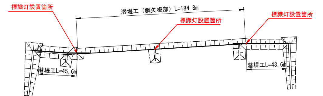
標識灯設置箇所位置図
