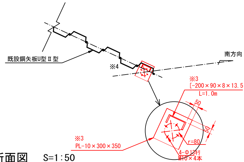
PL取付平面図 S=1:50
