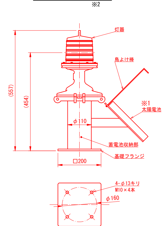
標識灯詳細図 S=1:10
