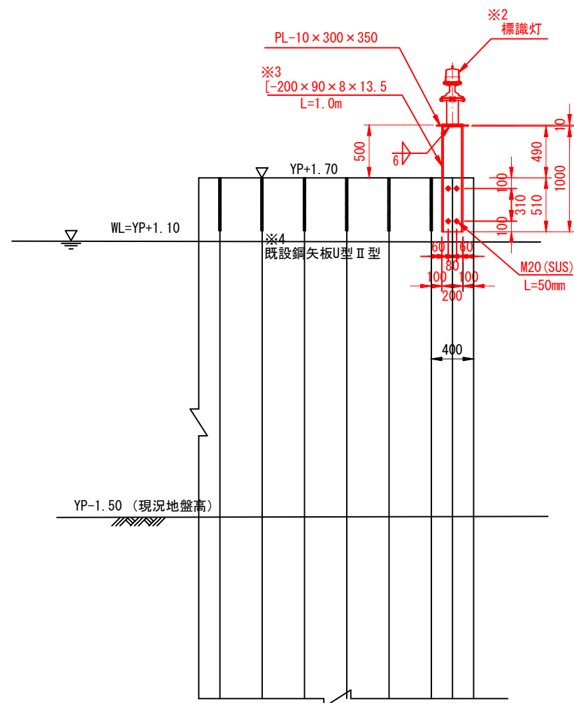
側面図 S=1:50
