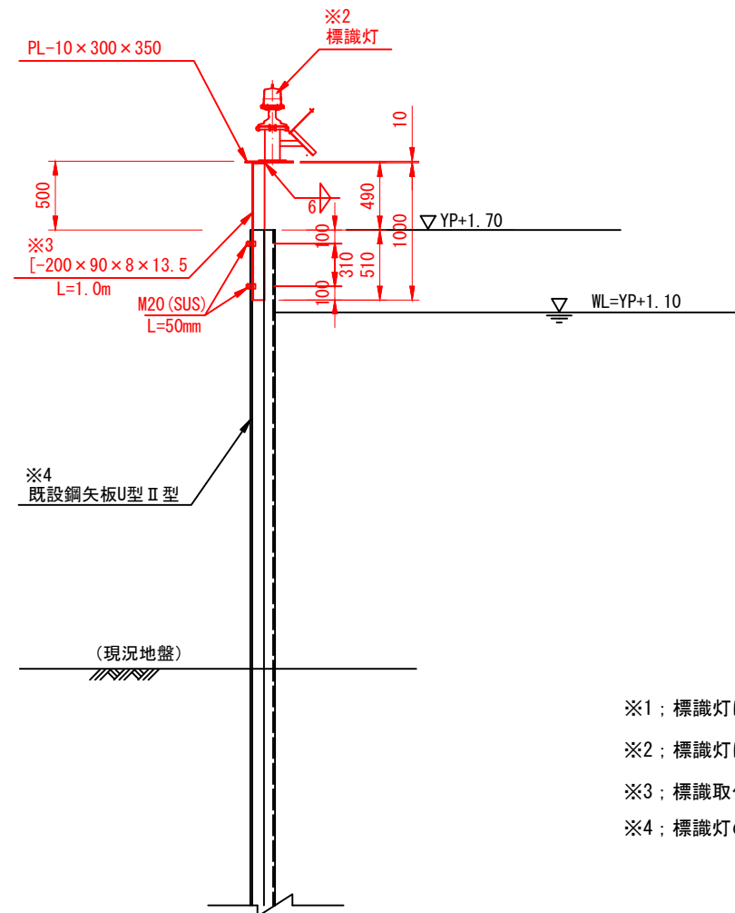
断面図 S=1:50
