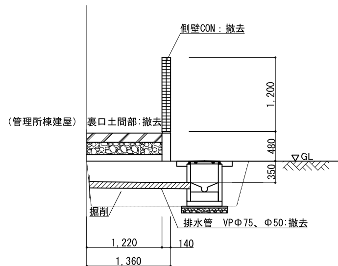
C-C断面図 S=1:30
