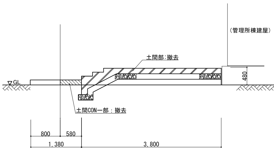
D-D断面図 S=1:30
