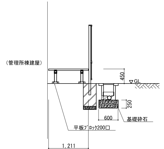
C-C断面図 S=1:30
