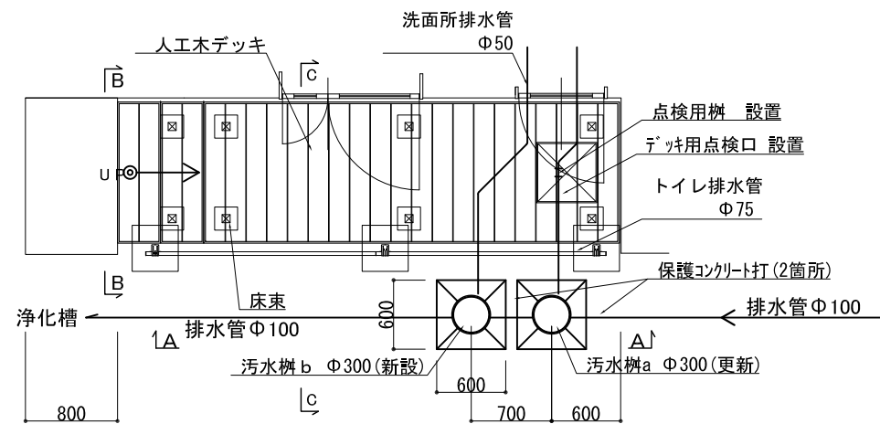
平面図 S=1:30
