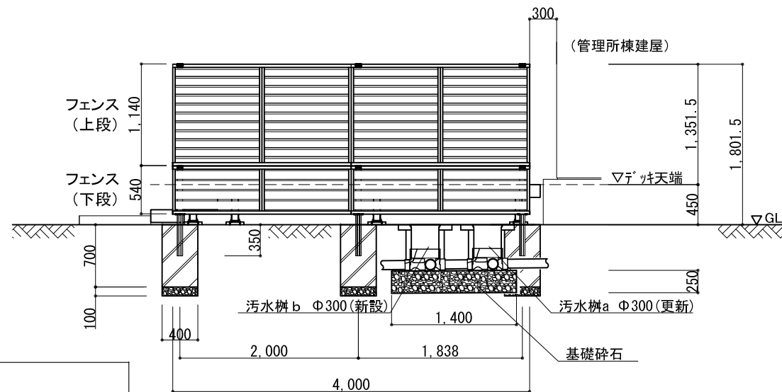
A-A断面図 S=1:30
