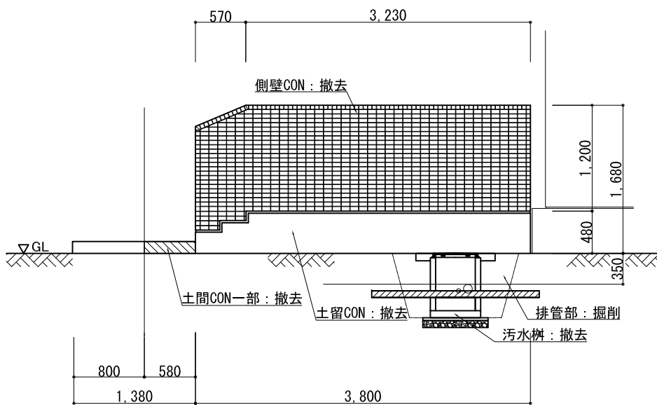
A-A断面図 S=1:30
