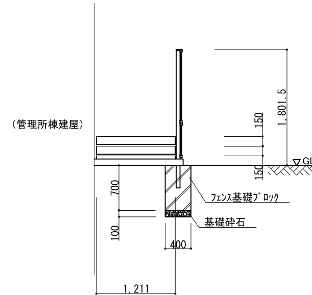
B-B断面図 S=1:30
