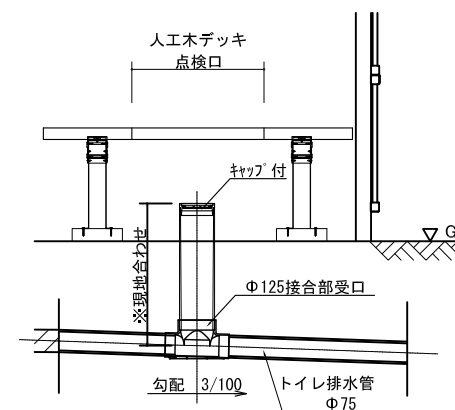
立上管部詳細図 S=1:15
