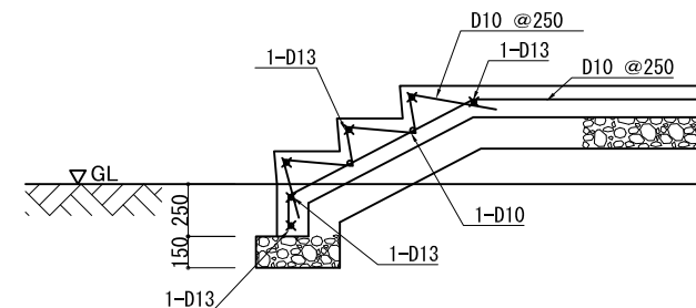
階段部断面図 S=1:20
