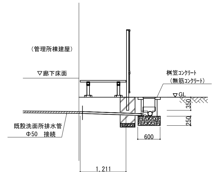
b 樹排水管敷設断面図 S=1:30
