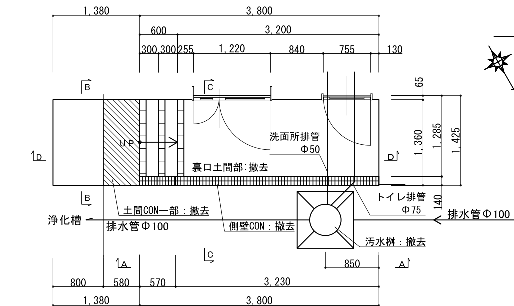
平面図 S=1:30
