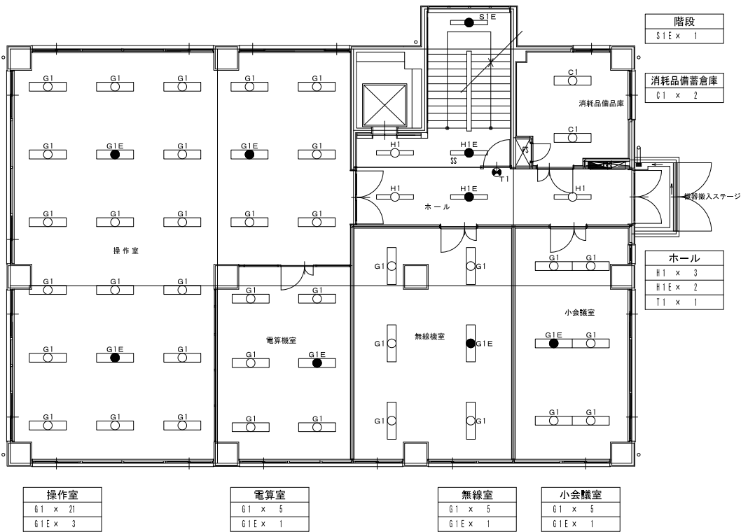
3階平面図
