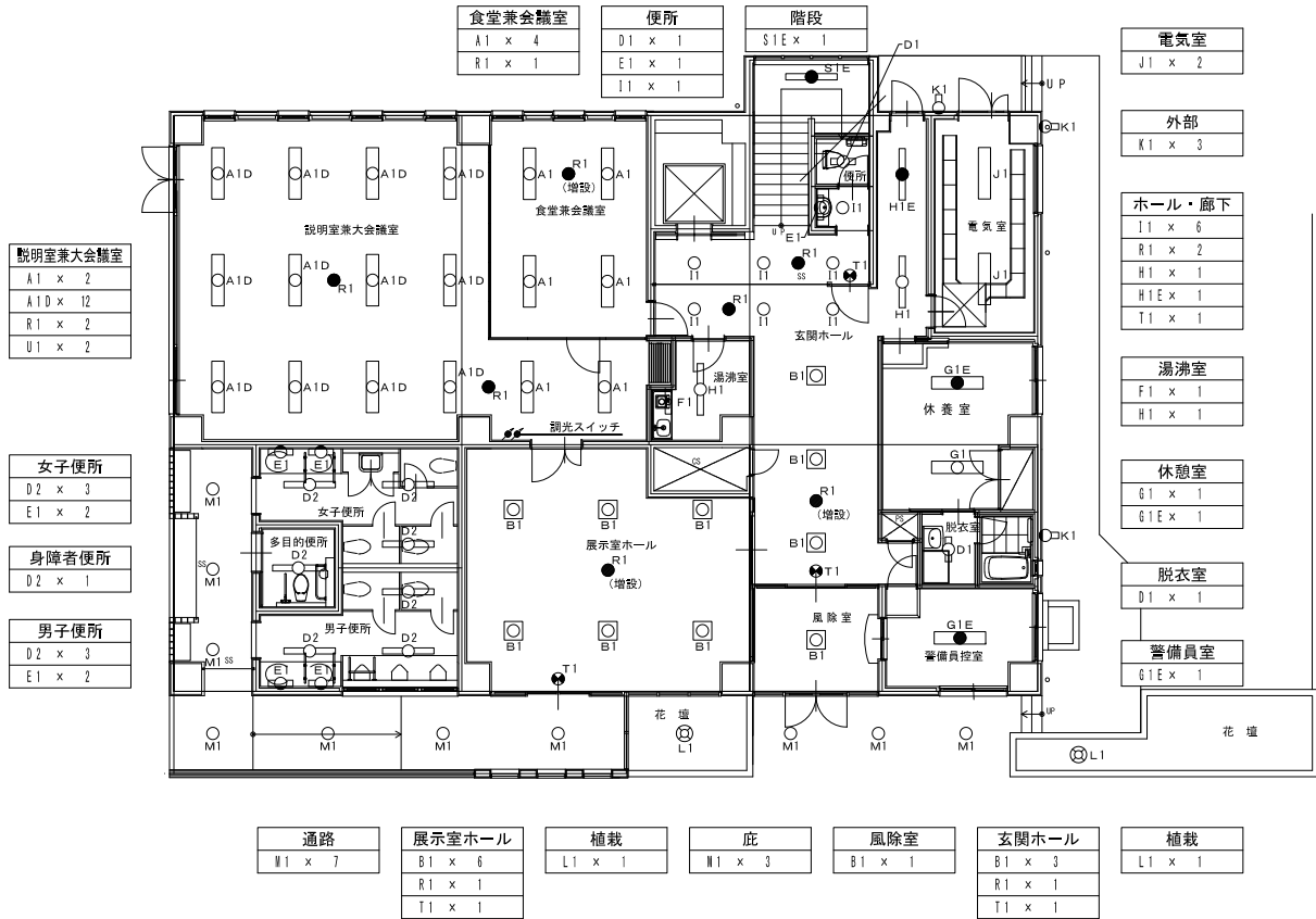
1階平面図
