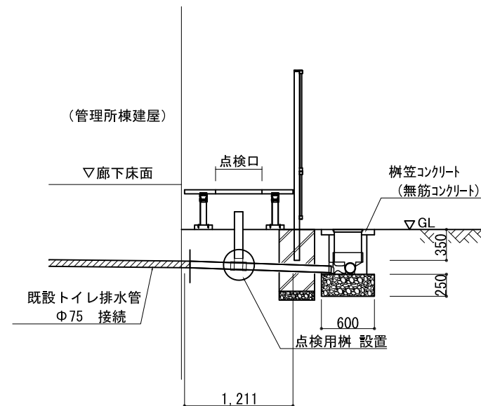
a 樹排水管敷設断面図 S=1:30
