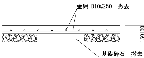
土間コンクリート断面図 S=1:20
