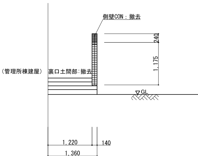
B-B断面図 S=1:30
