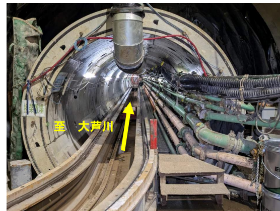
写真一 黒川導水路 起点側 (黒川流入立坑から撮影)
