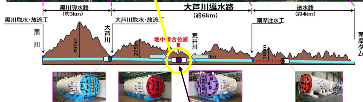
シールドマシン (トンネルを掘る機械)
