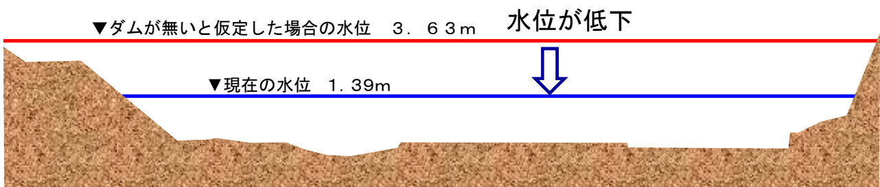
図2 下久保ダムにより想定される水位の低減（八塩橋付近）
