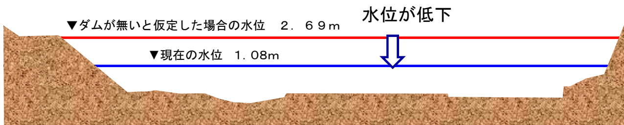
図2 下久保ダムにより想定される水位の低減（八塩橋付近）
