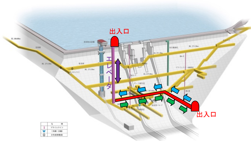
背面透視図
