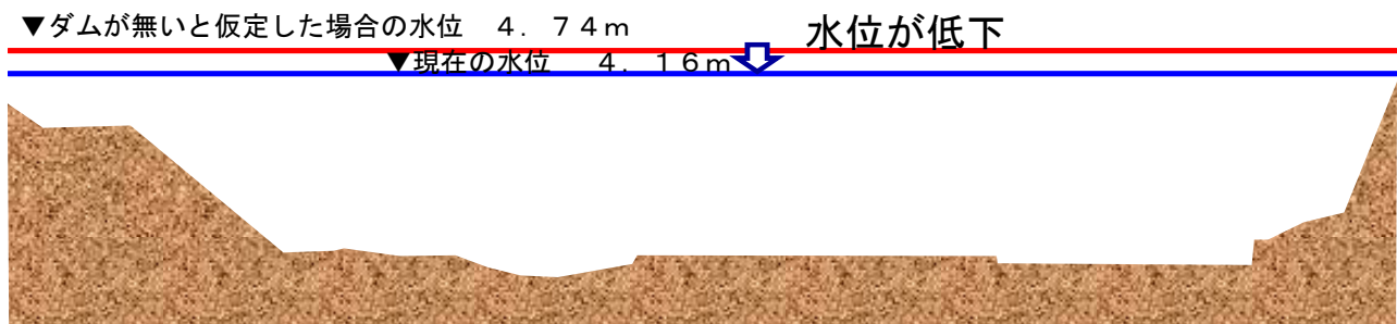
図2 下久保ダムにより想定される水位の低減（八塩橋付近）
