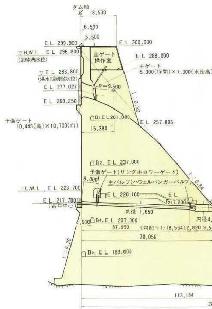
標準断面図(1)
