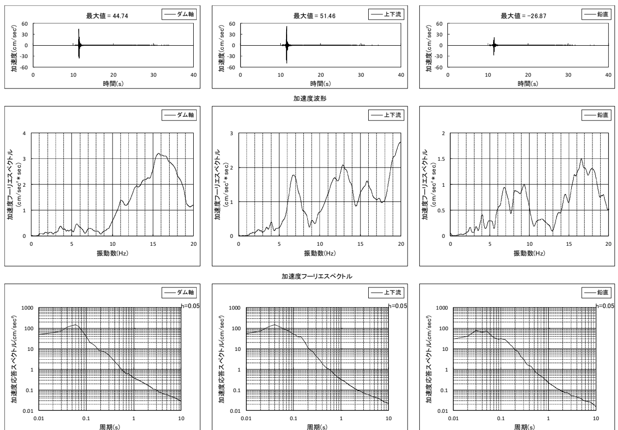
加速度応答スペクトル 〇〇ダム地震観測記録(yyyy年xx月xx日xx時xx分) 下部監査廊
