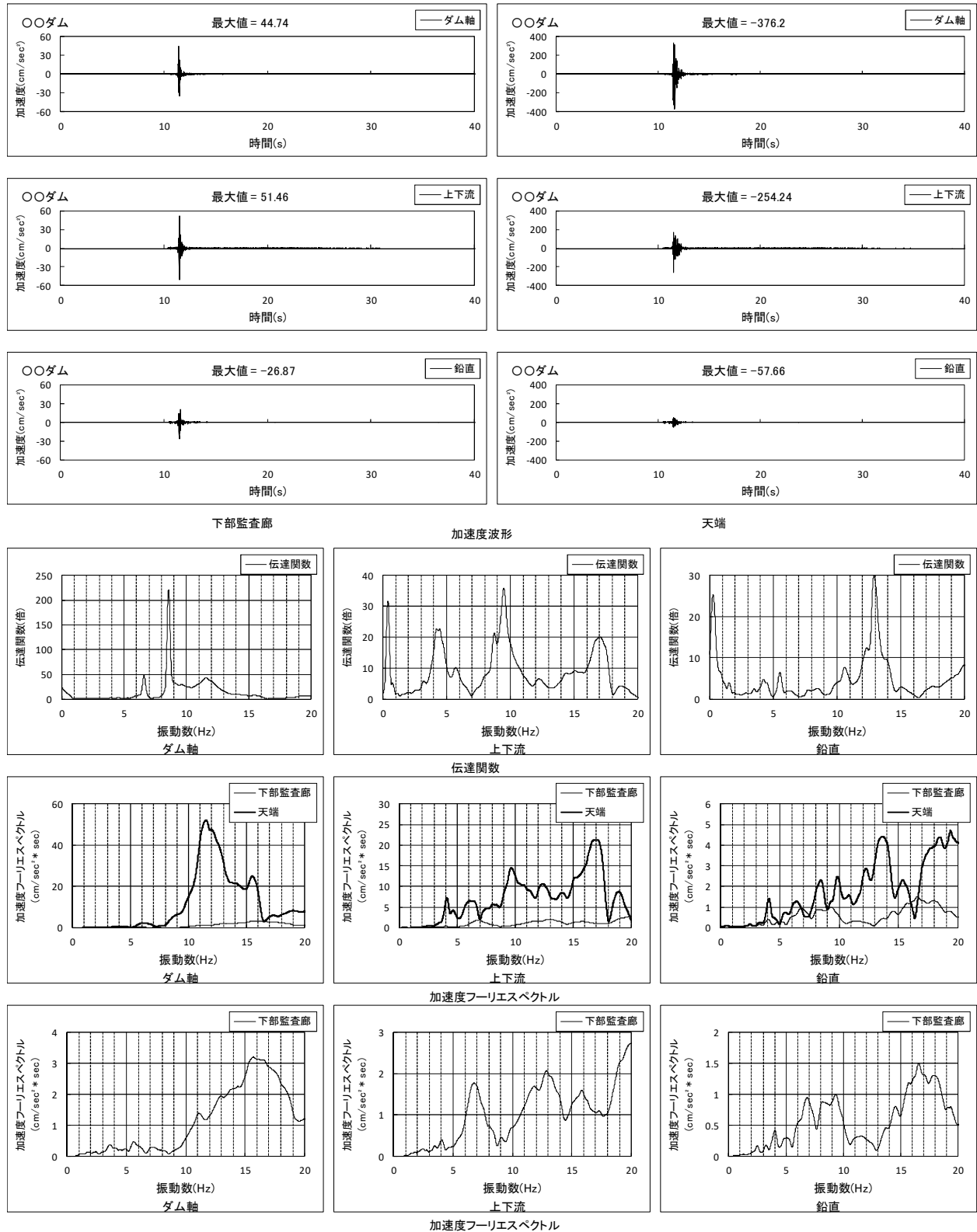
図 2(2) 〇〇ダム 観測記録 (xxxx 年 xx 月 xx 日 00 時 00 分) 基線補正後
