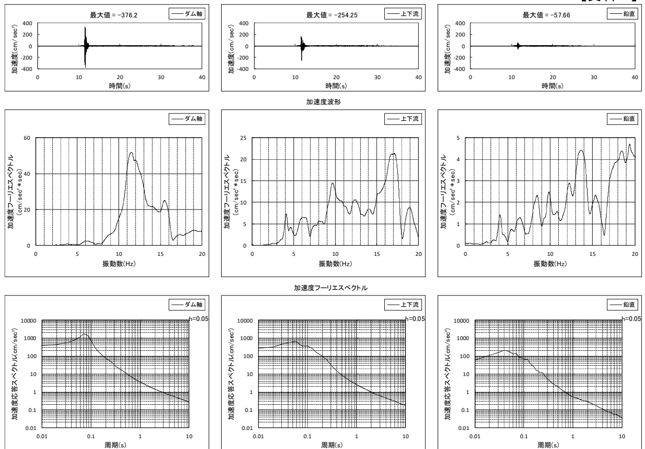
加速度応答スペクトル 〇〇ダム 地震観測記録(XXXX年XX月XX日〇〇時〇〇分) 天端
