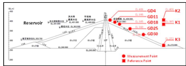
GPS 計測位置断面図 (赤丸箇所)
