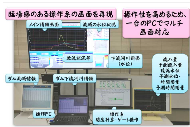
ダム防災操作訓練シミュレータのマルチ画面
