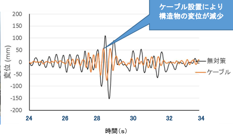
無対策とケーブル設置後の構造物の変位比較（解析結果）
