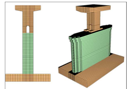
2次元非線形FEM解析モデル図
