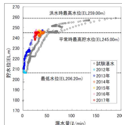
貯水位と漏水量の相関図の例
