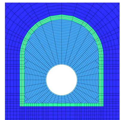
内挿鋼管(エアミルク充填)のトンネル断面のモデル例
