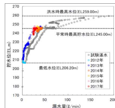
貯水位と漏水量の相関図の例
