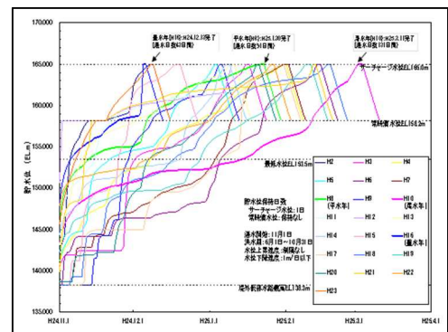
試験湛水シミュレーション図
