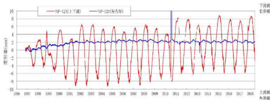
コンクリートダム堤体変形の例（プラムライン計測結果）
