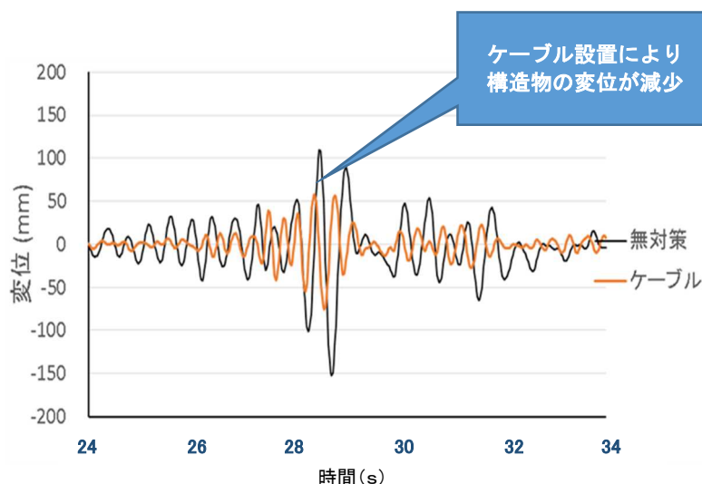
無対策とケーブル設置後の構造物の変位比較（解析結果）
