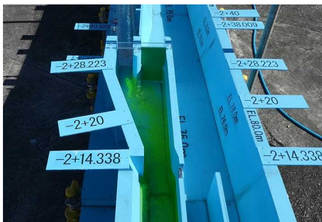
水理模型実験状況
