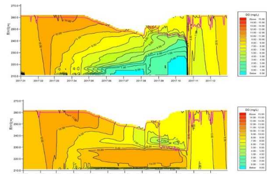
川上ダムにおけるDO(溶存酸素)予測 (上) 深層曝気無し、(下) 深層曝気有り
