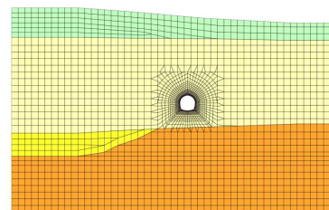
山岳工法トンネル断面のモデル例
