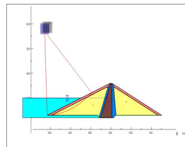
フィルダム堤体の安定計算
