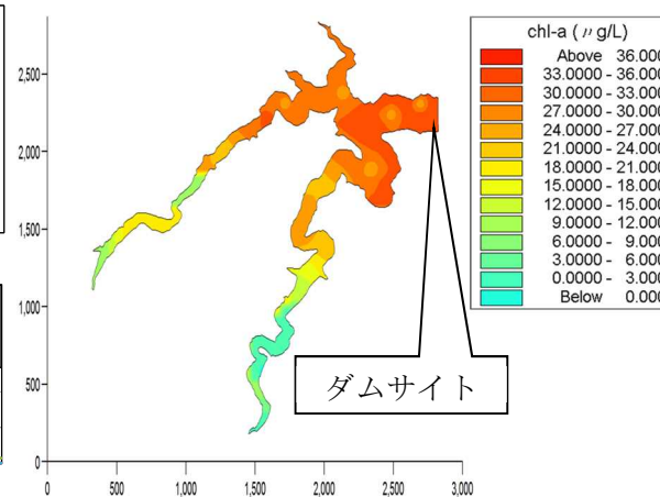
クロロフィル a の計算結果（平面図）
