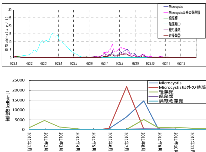
上図：藻類別の計算結果（ダムサイト地点）
