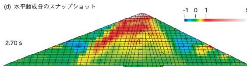
数値解析結果 (FEM モデル)
