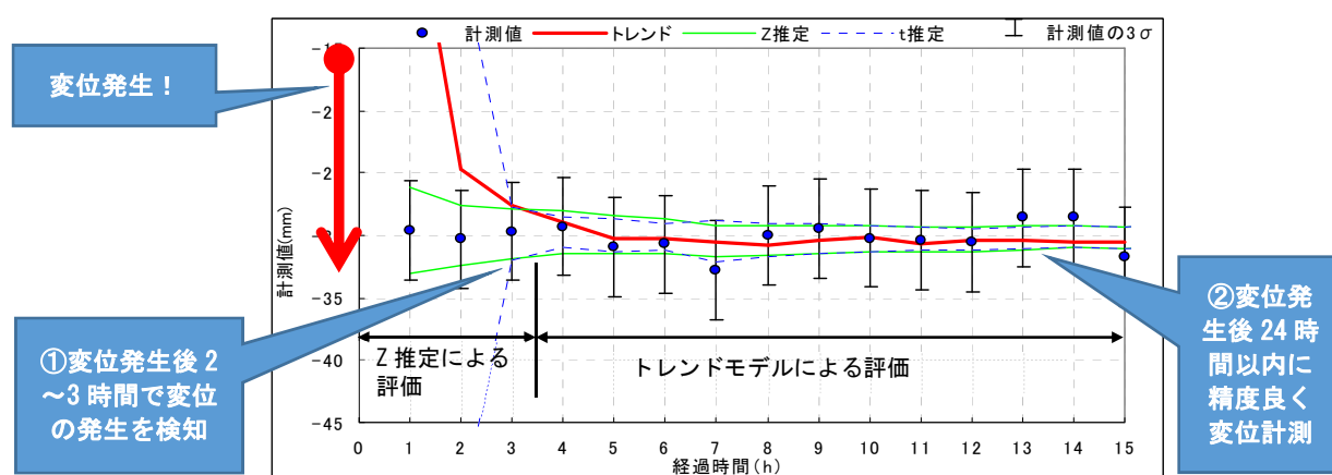
30mm の突発的な変位が発生した場合の検討図
