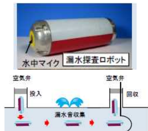
漏水探査ロボットによる管路診断
