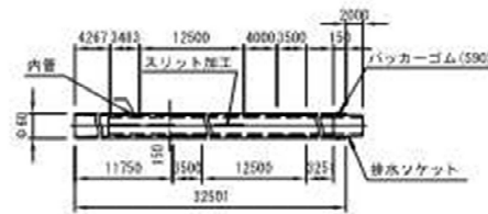
スリット加工、排水ソケット、内管付 VP50
