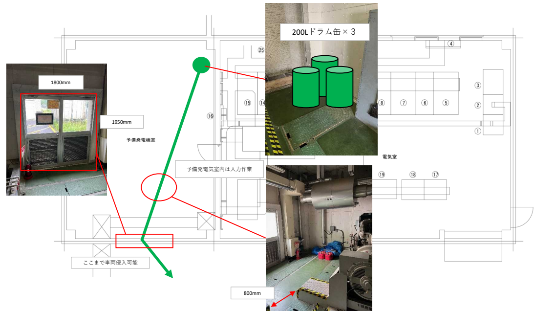
受配電棟 1F平面図
