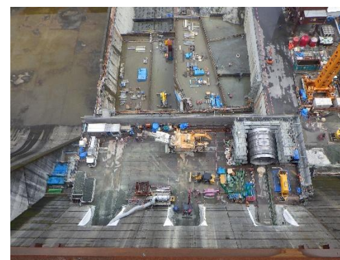
放流管設置中(令和7年8月)
