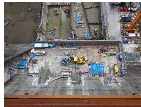
放流管設置中(令和7年9月)
