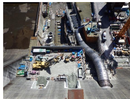
放流管設置中(令和8年3月)
