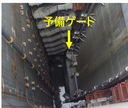
上流仮締切上流側から見た予備ゲート
