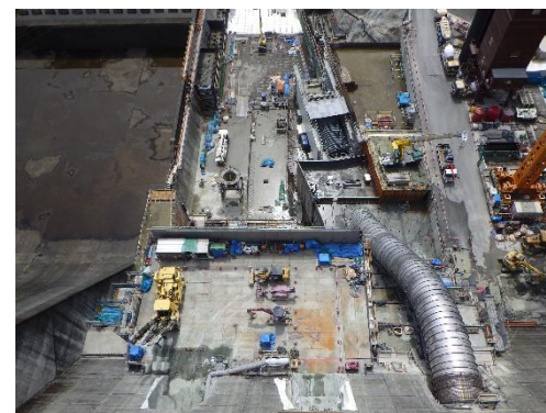
放流管設置中(令和8年4月)
