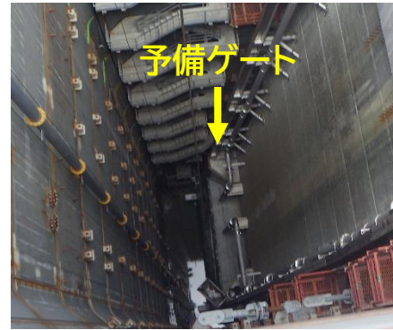
上流仮締切上流側から見た予備ゲート
