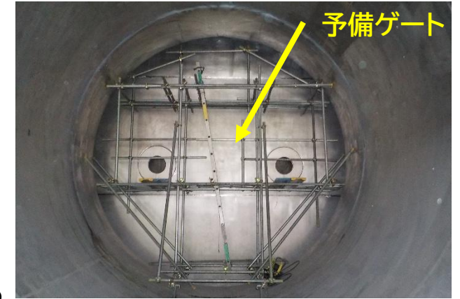
3号放流管下流側から見た予備ゲート
