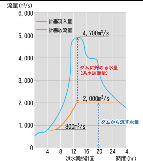
洪水調節計画図(※変更なし)
