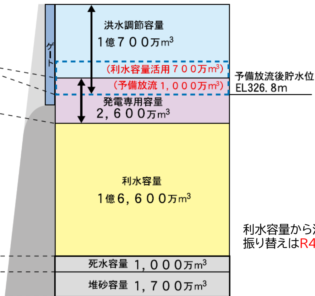
ダム再生事業後
