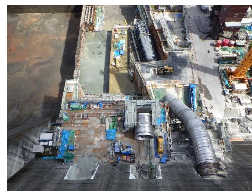
放流管設置中(令和8年8月)
