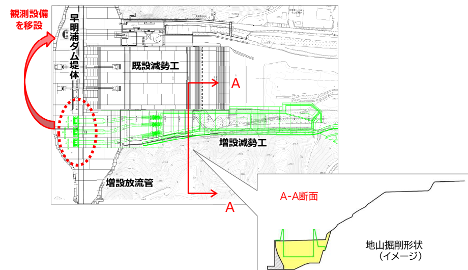
【平面配置見直し後】
