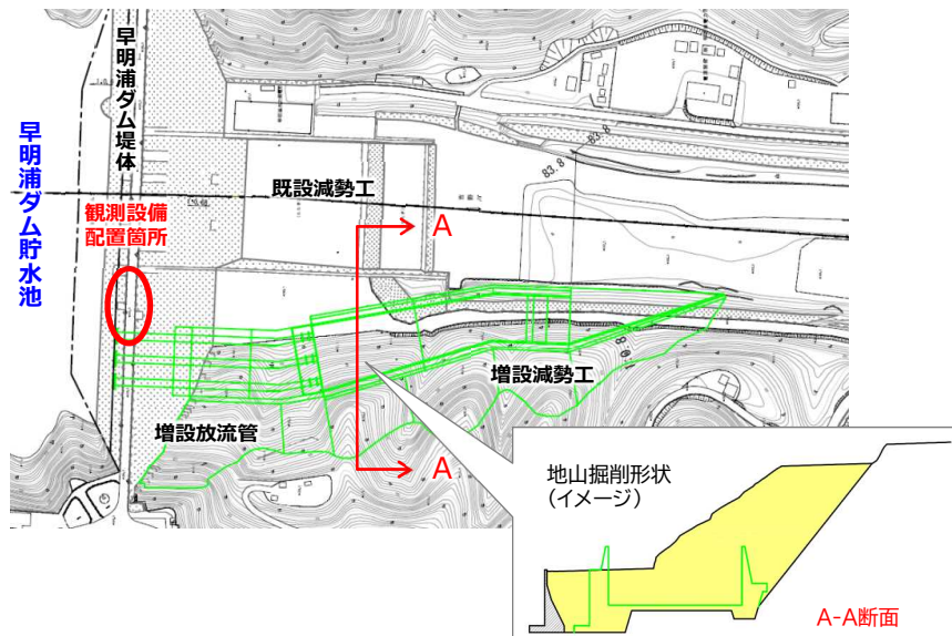
【平面配置見直し前(原設計)】
