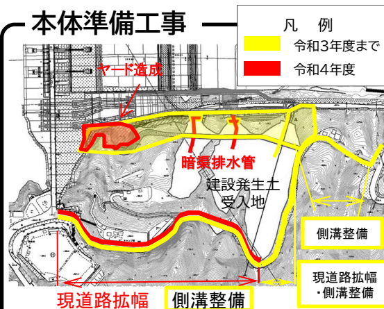
工事用道路整備状況
