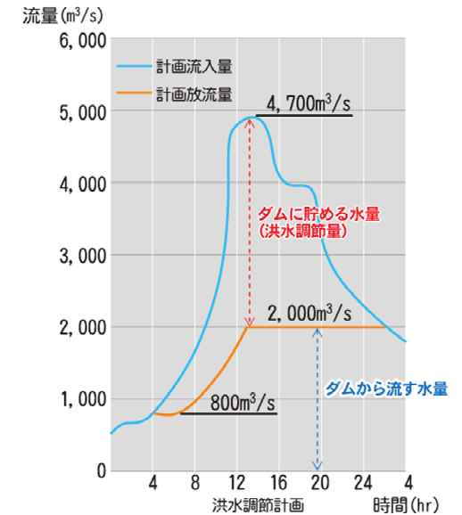
洪水調節計画図
