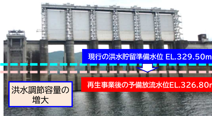
クレストゲートと洪水貯留準備水位の関係
